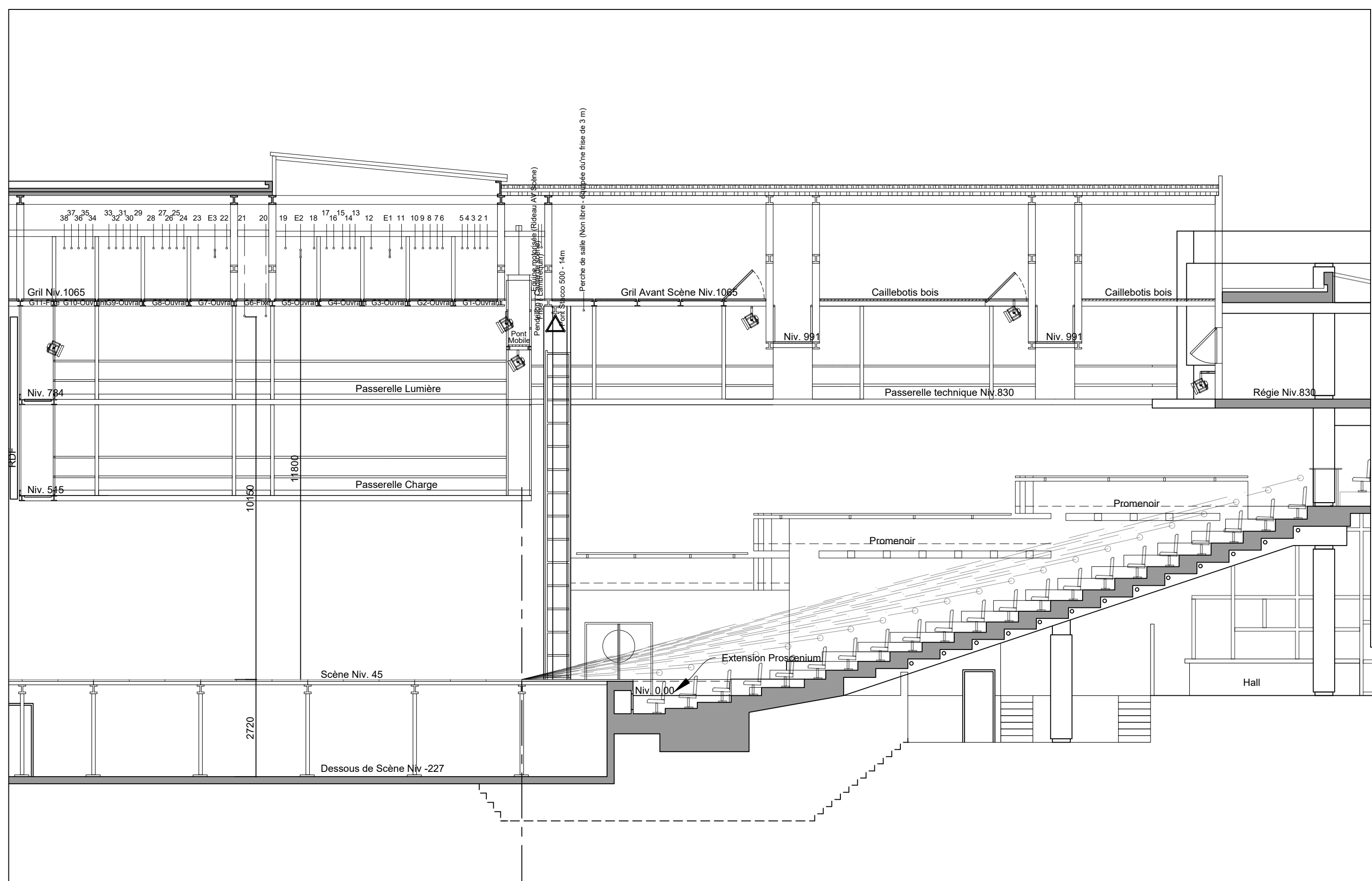
Coupe Longitudinale Grande Salle
